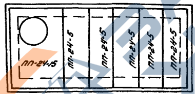
Схема перекрытия
