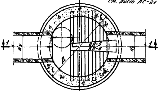
План-разрез по осям труб
