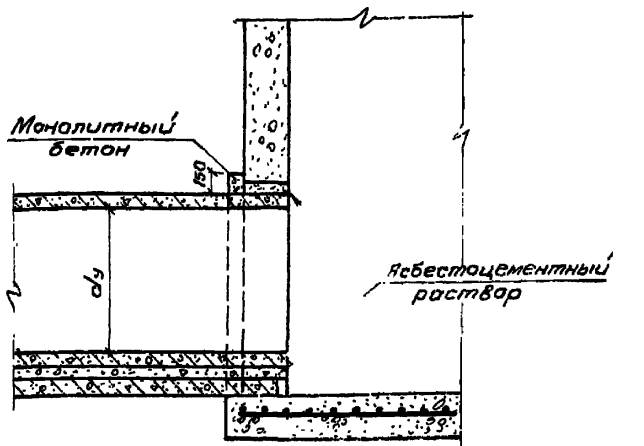
Заделка труб в непрсадачных сухих грунтах
