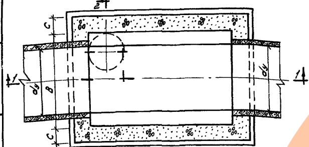
План (разрез по осм труб) Колодцы для непросадочных грунтов К-1
