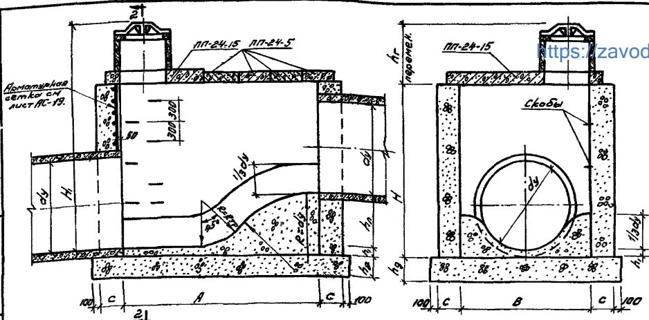
Разрез 1-1
