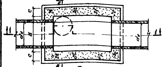
План (разрез по осям труб)
