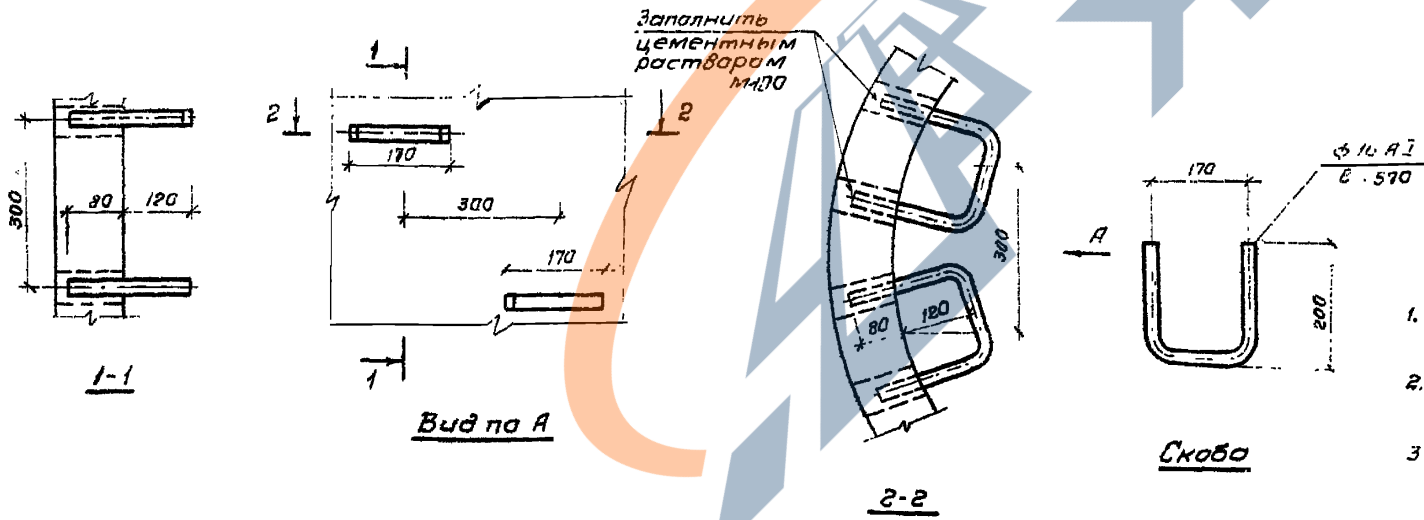
Выборка материала на 1 скобу
