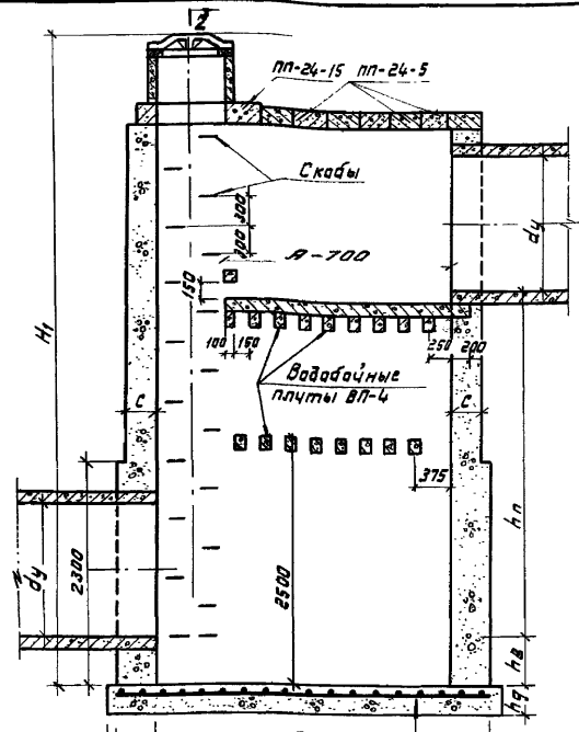
Разрез 1-1
