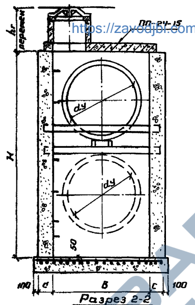
Разрез 2-2
