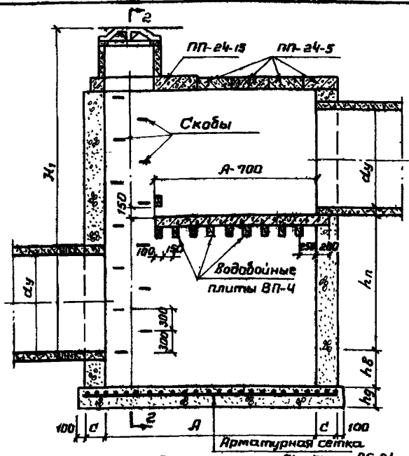
Разрез 1-1 ст. лист АС-21
