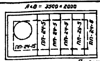
Схемы перекрытий
