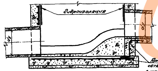
Разрез 1-1 Колодцы для просадочных грунтов К-2
