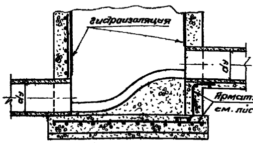
Разрез 1-1
