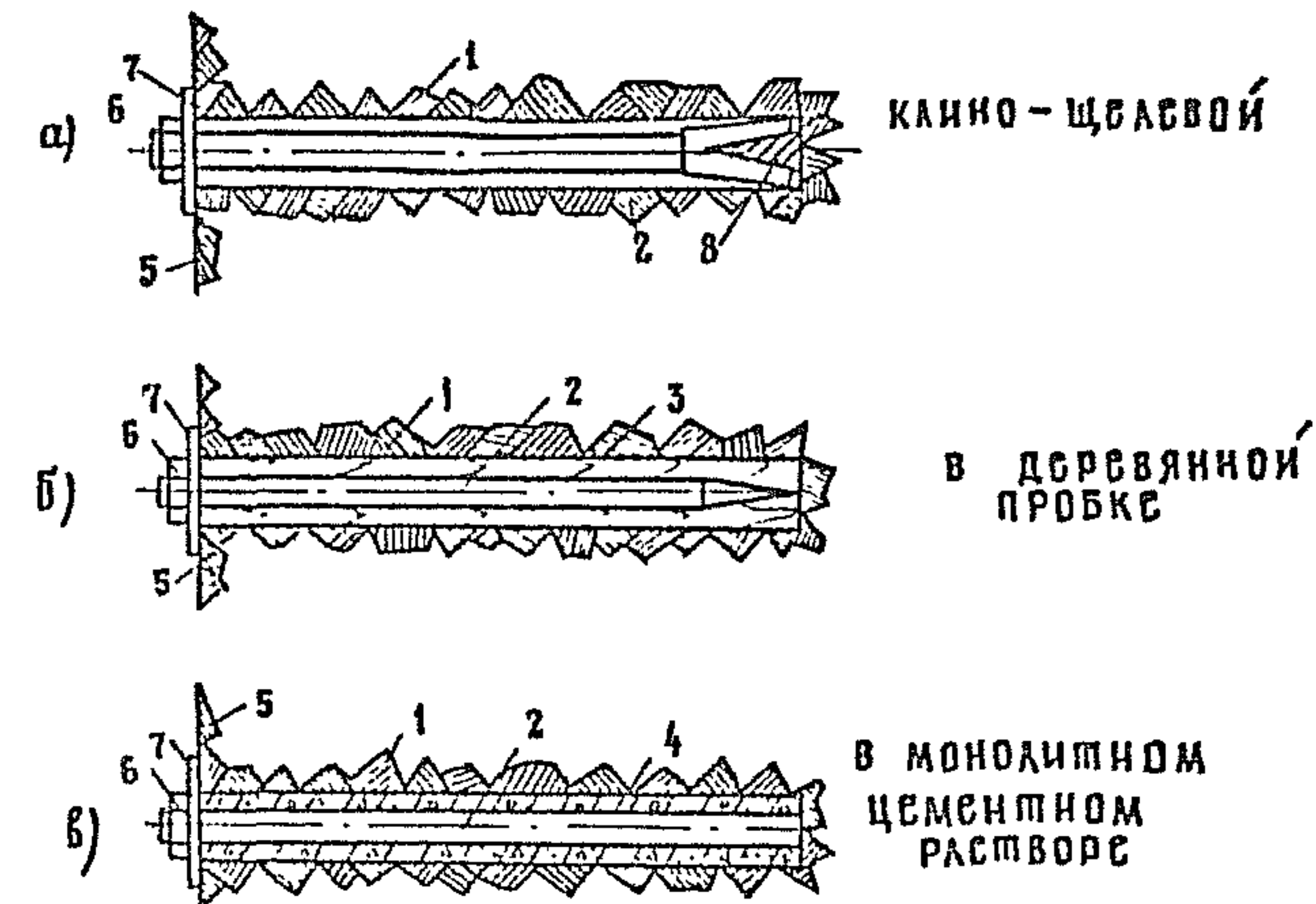
ПРИМЕРЫ ЗАДЕЛКИ АНКЕРОВ
