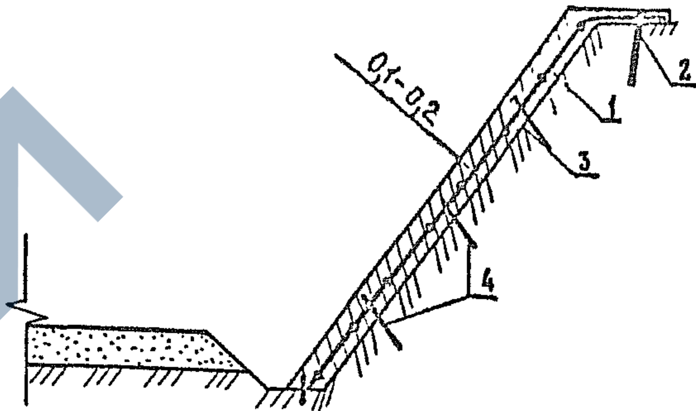
ПРИМЕРЫ ЗАДЕЛКИ АНКЕРОВ
