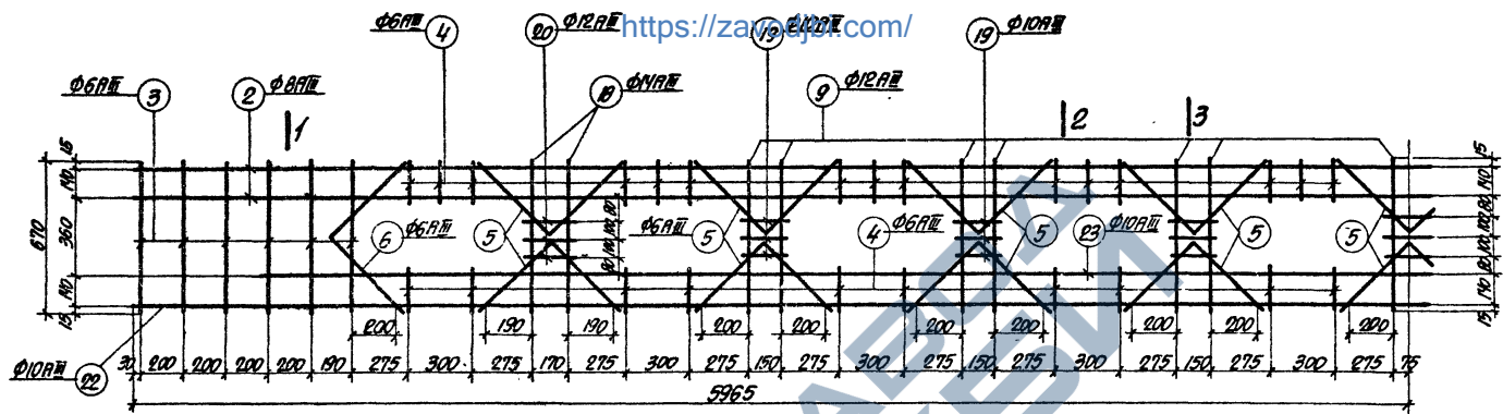
КАРКАС КР-2
