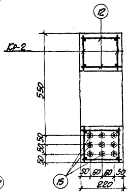
2-2 ДЛЯ БАЛОК Б-2П-а,б,в
