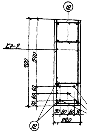
1-1 ДЛЯ Б-20V-а,б,в
