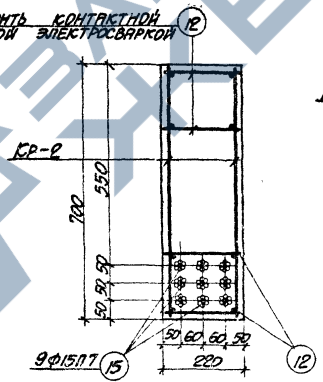
1-1 ДЛЯ БАЛОК Б-2П-а,б,в
