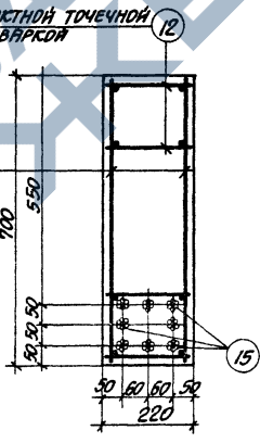
1-1 ДЛЯ БЛОК Б-1П-а,б,в
