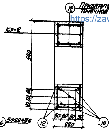
2-2 ДЛЯ Б-20B-а,б,в
