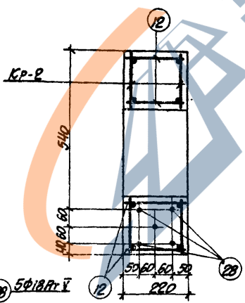
2-2 ДЛЯ Б-20V-а,б,в
