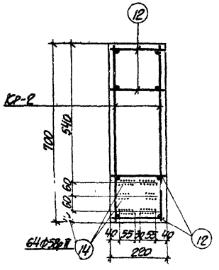
1-1 ДЛЯ БАЛОК Б-2ВрII-а,б,в
