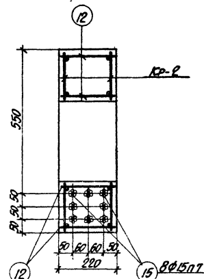
2-2 ДЛЯ БЛОК Б-1П-а,б,в
