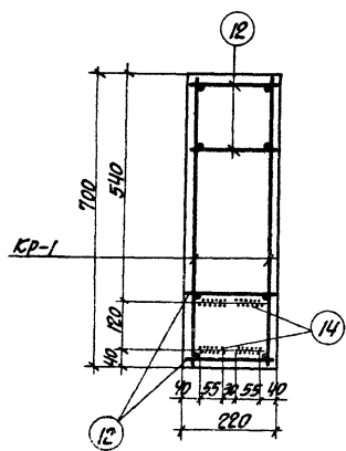
1-1 ДЛЯ БЛОК Б-1ВрII-а,б,в
