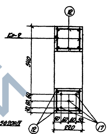
2-2 ДЛЯ Б-20IV-а,б,в
