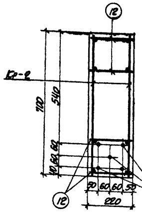
1-1 ДЛЯ Б-20B-а,б,в
