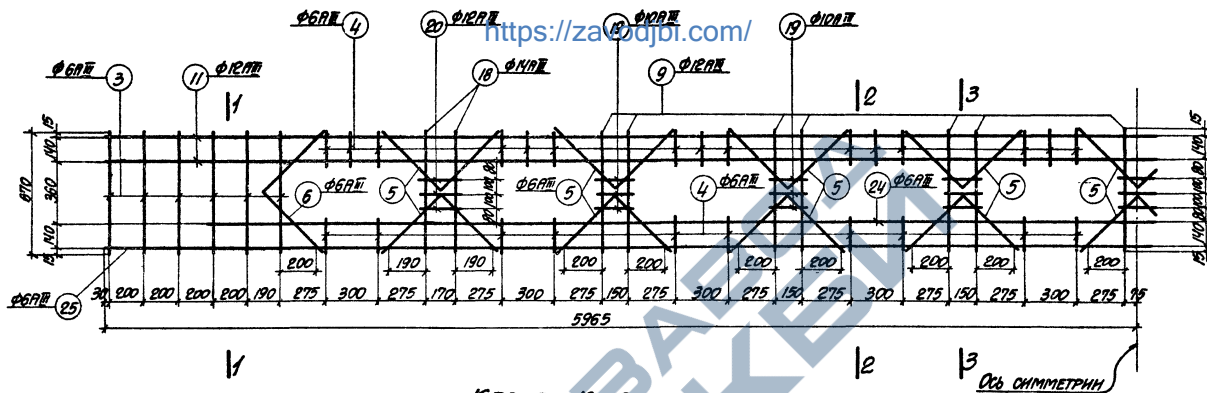
КАРКАС КР-3
